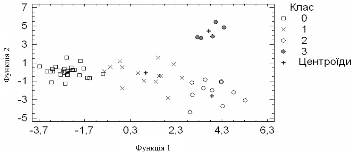
Рис. 3. Графіки дискримінантних функцій за результатами аналізу клініко - лабораторних показників хворих на поєднану патологію
